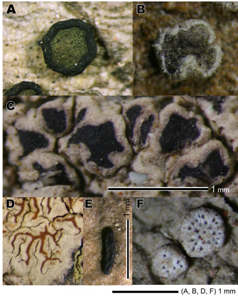
Fig. 1. 日本産リトマスゴケ科の多様な子器。 A, レキデア型裸子器。 B, レカノラ型裸子器。 C-E, リレラ。 F, 被子器 (ストロマ)。 A, Cresponea macrocarpoides ; B, Roccellina niponica ; C, Graphidastra japonica ; D, Enterographa anguinella ; E, Opegrapha varia ; F, Dichosporidium boschianum . (乾燥標本)。
